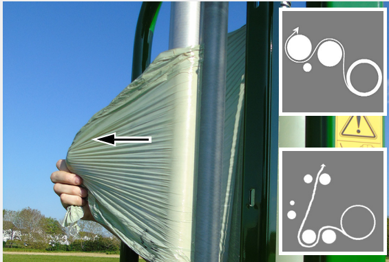
Banen til nedre forstrekker
