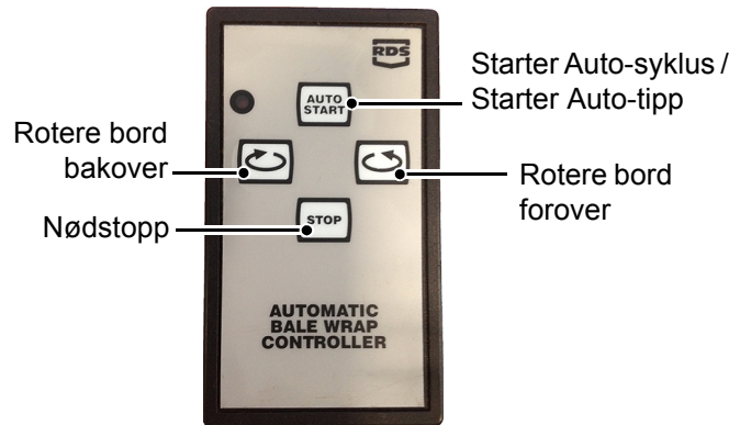
Infrarød fjernstyring
