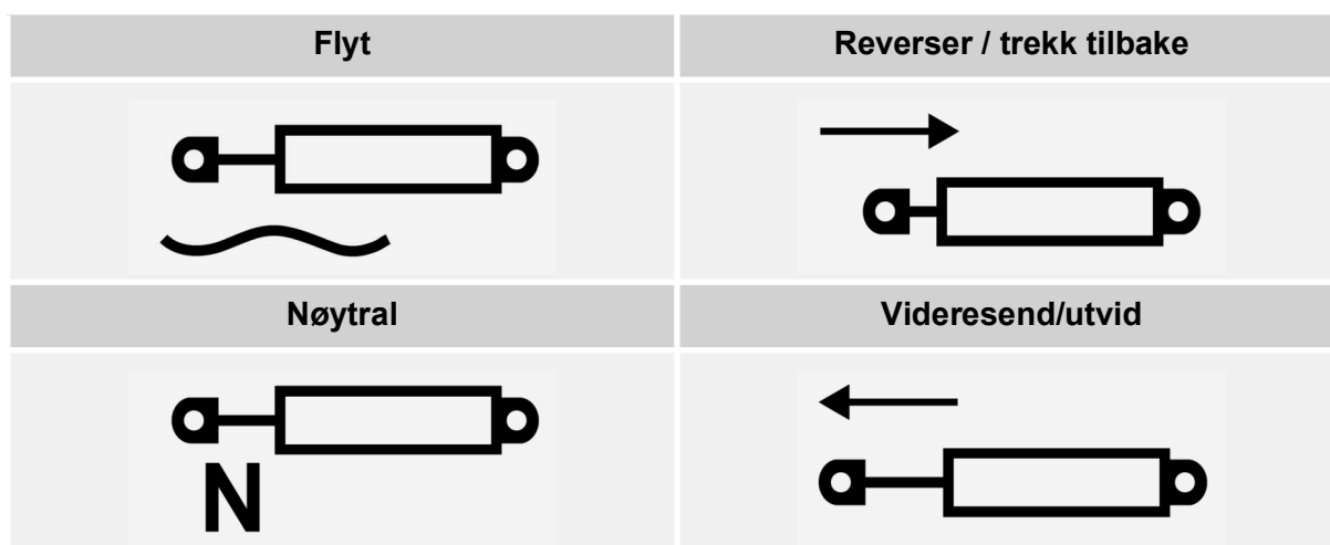
Hydrauliske kontrollfunksjoner
